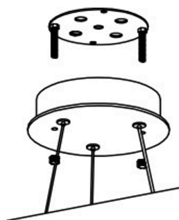
1. Открутите гайки и снимите планку.
