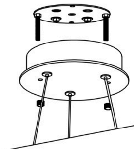
5. Закрутите декоративные болты.
